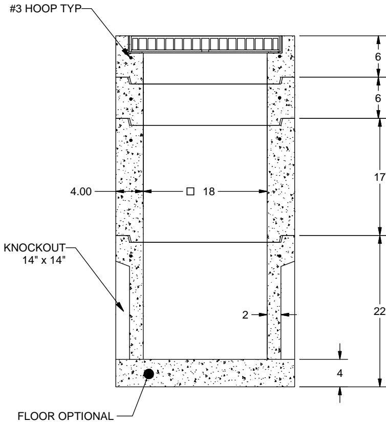
SECTION A-A
